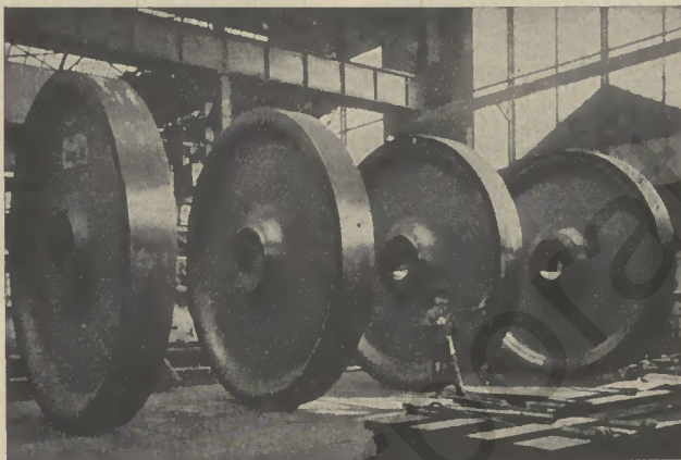
Stahlguß-Allgemeiner Schwungräder von 4400 mm Ø
