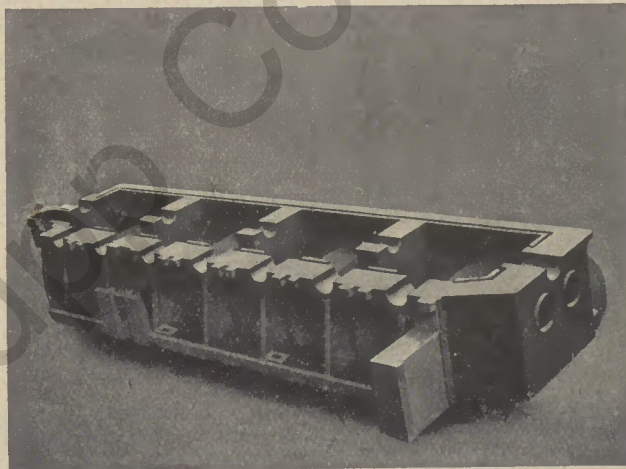
Rollgangrahmen aus Stahlguß im Gewicht von ca. 15 150 Kilogramm
