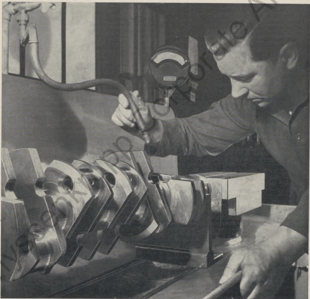
Oberflächenprüfung einer fertigen Kurbelwelle nach dem Magnetpulververfahren, Werk Hemscheid
