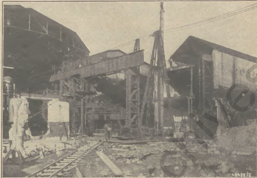
Bild 3: Montage des Kranbahnträgers rechts mit Anschluß an die alte Hallenkonstruktion. Neben dem Kranbahnträger ist das Montagegerät sichtbar. Die Baugrube ist wegen Ueberdeckung nicht sichtbar
