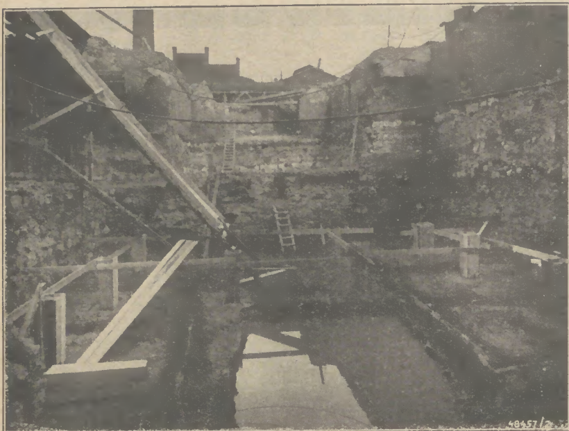
Bild 1: Die gewaltige Baugrube für die Presse. Im Vordergrund die Fundamentsohle, die kleinen Kästen dienen zur Aufnahme der Unterschrauben
