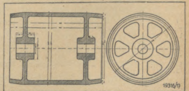
Bild 24: Facharbeit für Lehmformer: Gurttrommel (Aufgabe)
