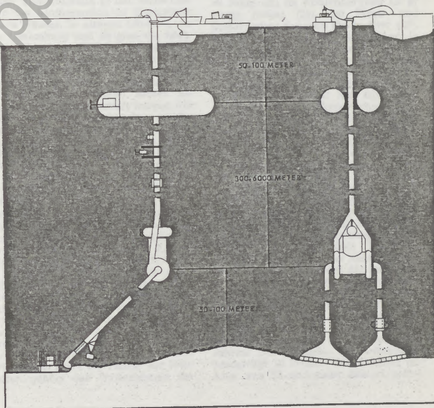
So stellen sich die Techniker die Hebung der Meeresschatze vor. Tief reichende Bagger saugen sie vom Meeresgrund an Bord eines Schiffes.
