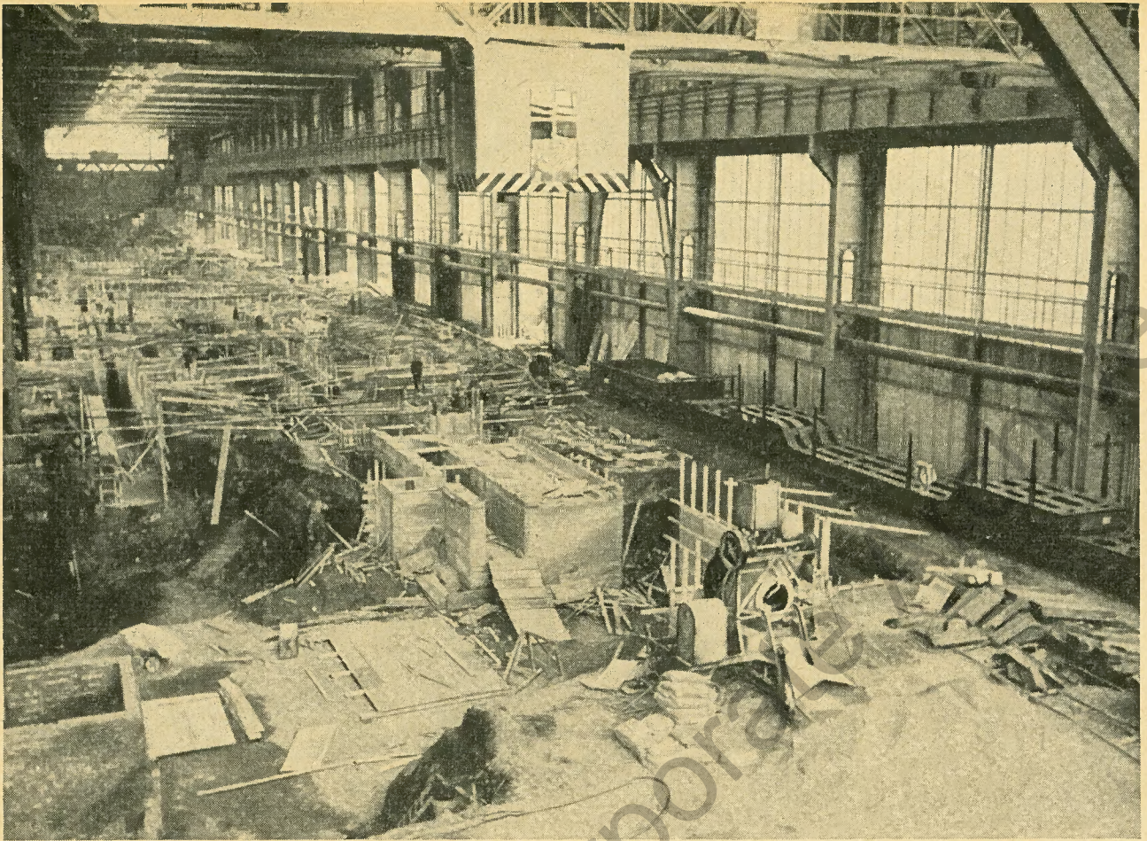
Blick in die Walzwerkshalle von Süden während des Baus der Maschinenfundamente
