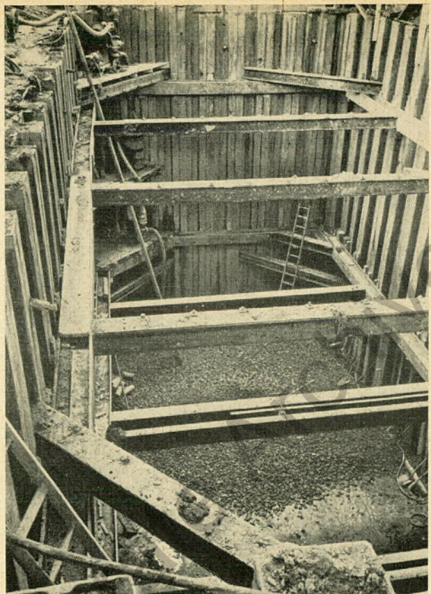
Ausgesteifter Spundkasten der Sintergrube (Staffel I)
