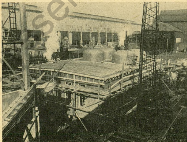
Pumpen und Filter der Wasserversorgung (im Hintergrund neue Walzwerkshalle)
