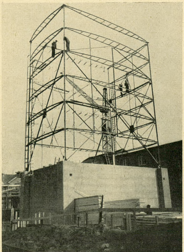
Kühlturm während der Montage
