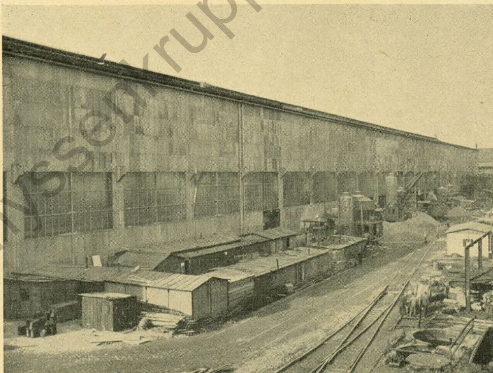
Blick gegen Ostwand der Walzwerkshalle mit der Baustelleneinrichtung
