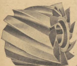
Walzenstirnfräser mit Spiralschneiden
