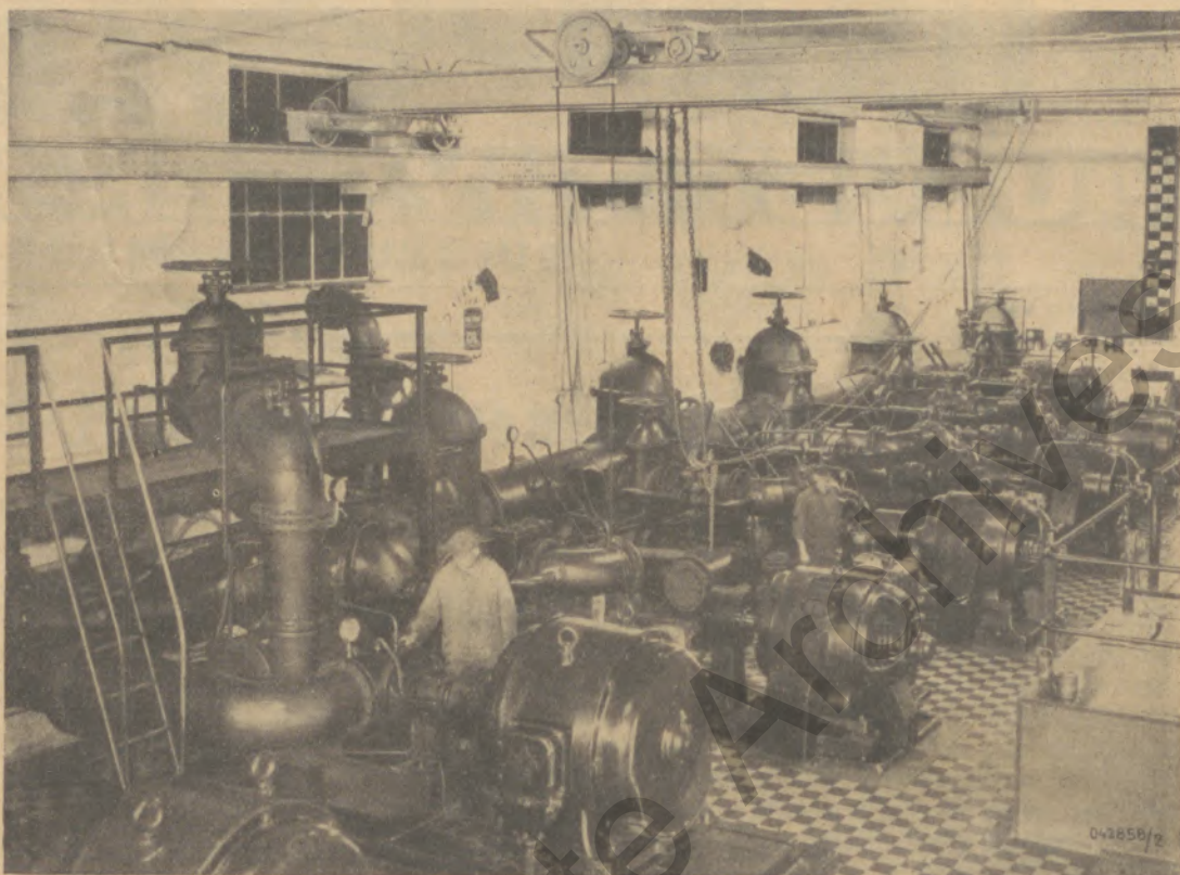
Die Pumpen mit Antriebsmotoren
