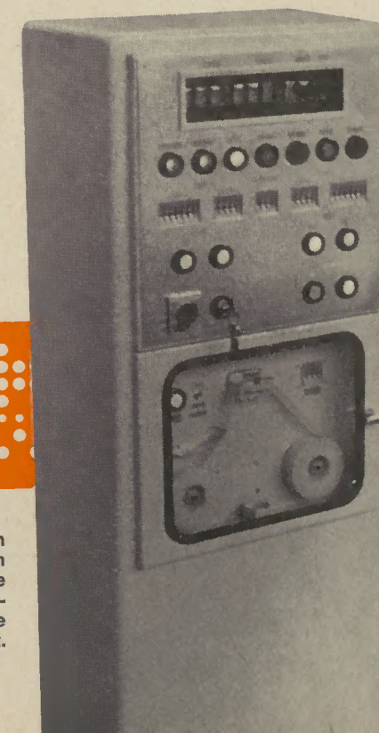
Der Lochstreifen wird in den neben der Maschine stehenden Schaltschrank für die Numerik eingelegt.
