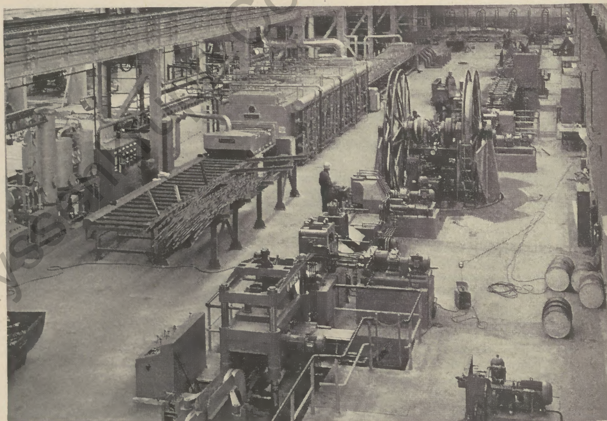
Die Produktionsanlage für geschweißte Qualitätsrohre
