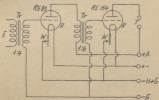
Abb. 1: Schema eines Verstärkers für Lautsprecherbetrieb.
