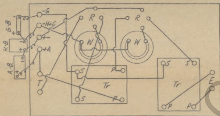
Abb. 2: Bauzeichnung des Verstärkers.
