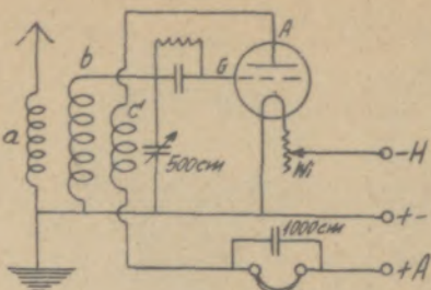
Abb. 3: Schaltbild eines Rückkopplungsempfängers.
