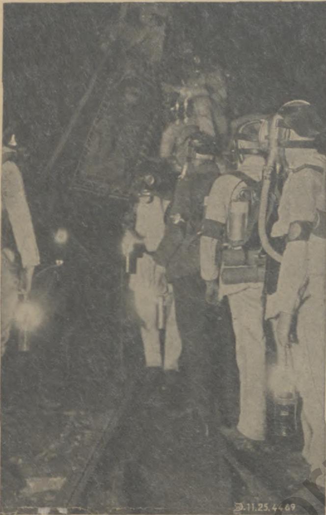
Verletzten-Transport mit Barczyk's Steiltransportbahre des Dräger-Werkes, Lübeck.
