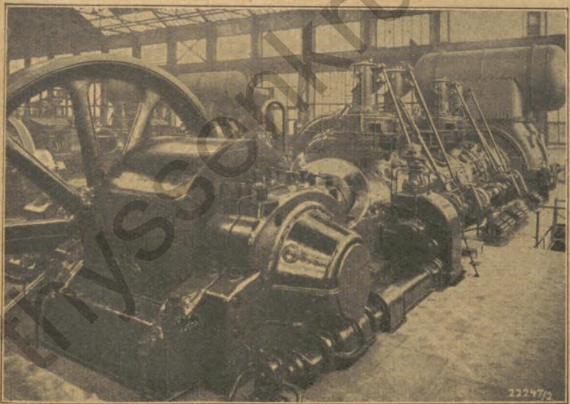
Gas-Gebläse C 6
