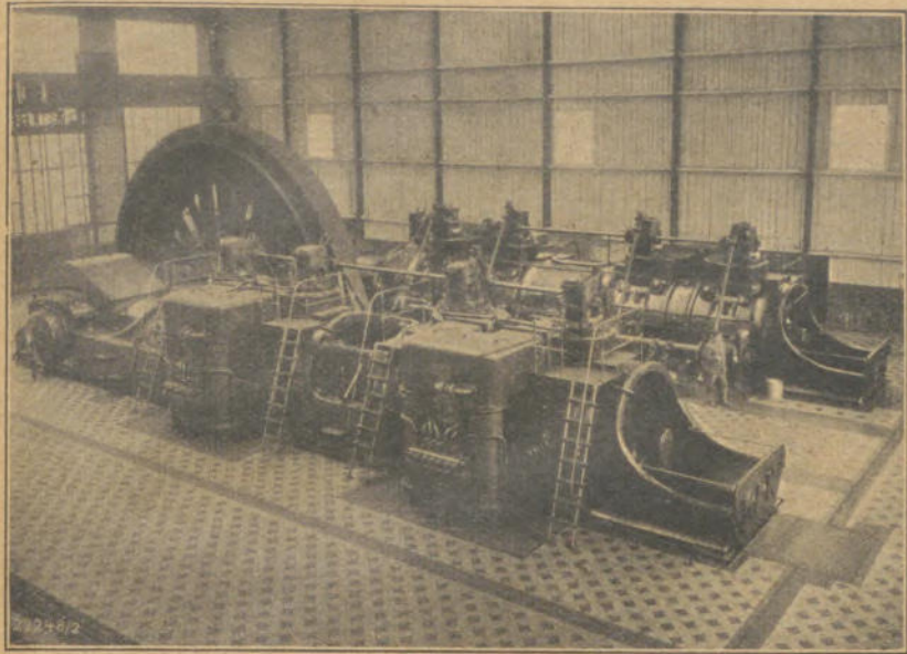
Gas-Dynamo C 5
