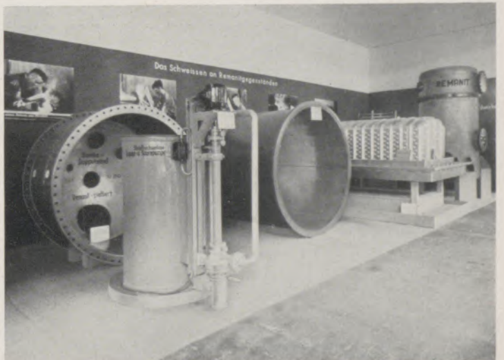
Remanit-plattierte Behälter
