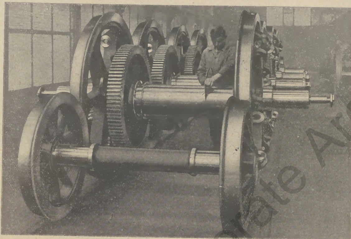
Eine Garnitur Radsätze für eine D o 1 - elektrische Lokomotive mit aufgezogenen Hohlwellen im Gewicht von 19.550 kg geliefert im Oktober 1927 für die A. E. G., Lokomotivfabrik, Hennigsdorf
