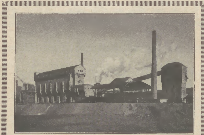
Koksereianlage Aufnahme von W. Benning, Hörde
