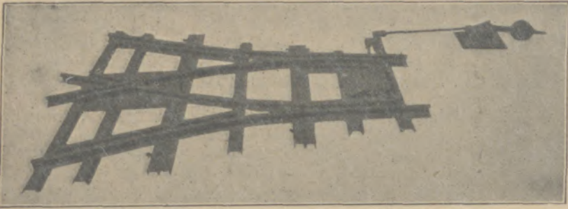
Bild 5: Zusammengebaute Weiche.
