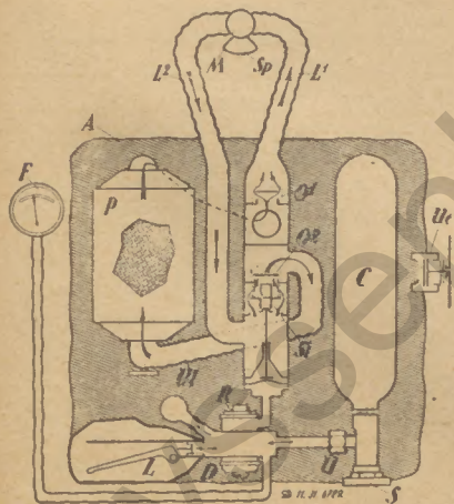
Abb. 2: Schnitt durch das Draeger-Alein-Gaschutzgerät, Modell 1931
