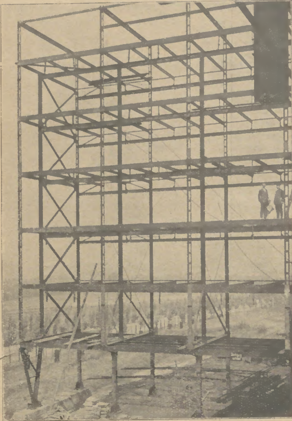
Durchblick durch das Stahlskelett des Haupttraktes
