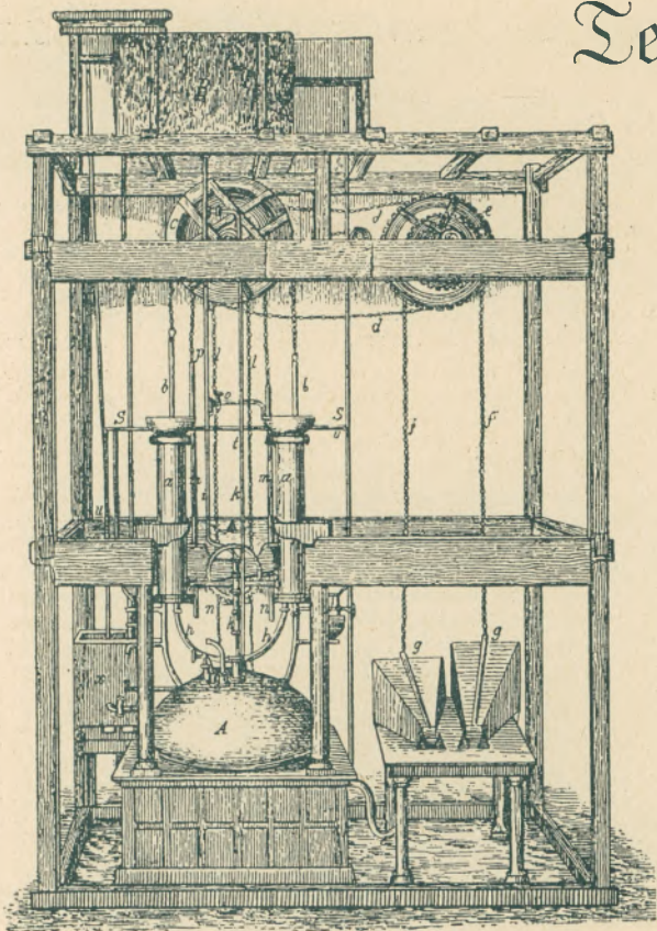
Die Polzunowsche atmosphärische Dampfmaschine, erbaut in Sibirien 1763 bis 1766.
