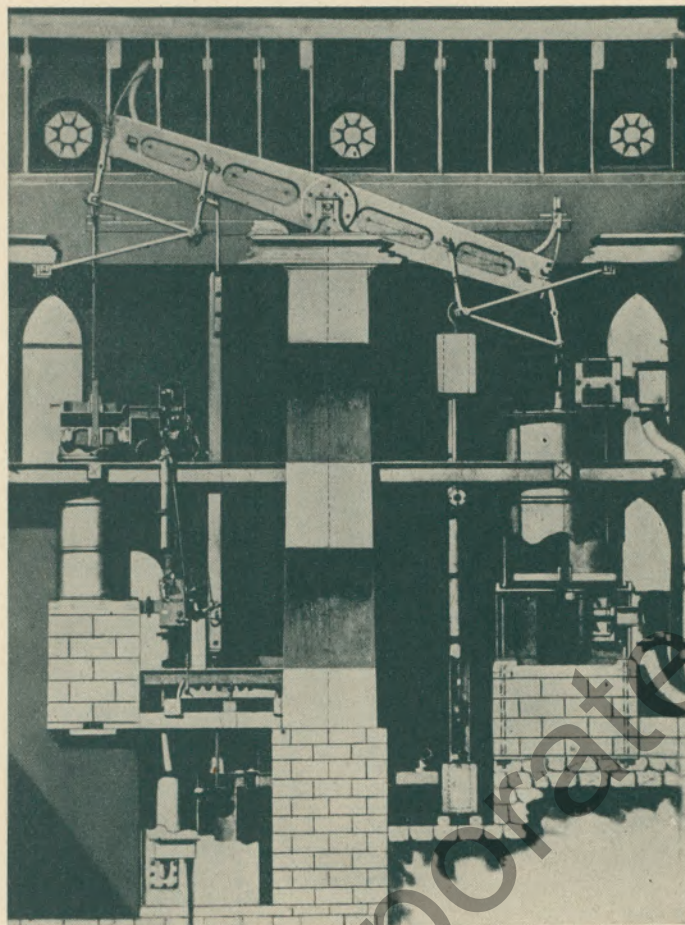
Dampfgebläse der Königshütte, von Holzhausen erbaut (1802).
