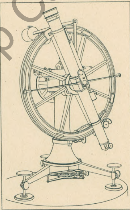
Reichenbachs großer astronomischer Kreis,
