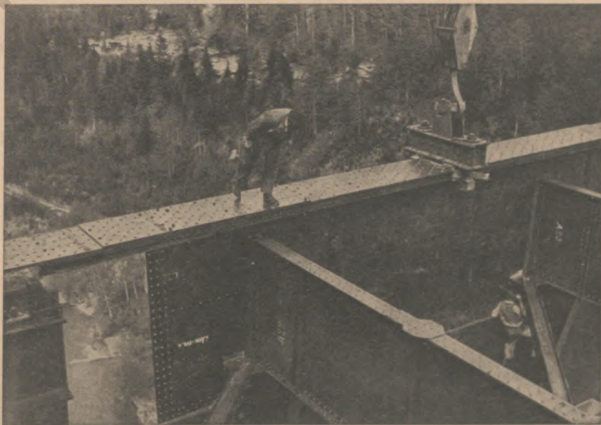
Montieren der Hauptträger, eine gefährvolle Arbeit, bei der Schwindel- freiheit unerlässlich ist
