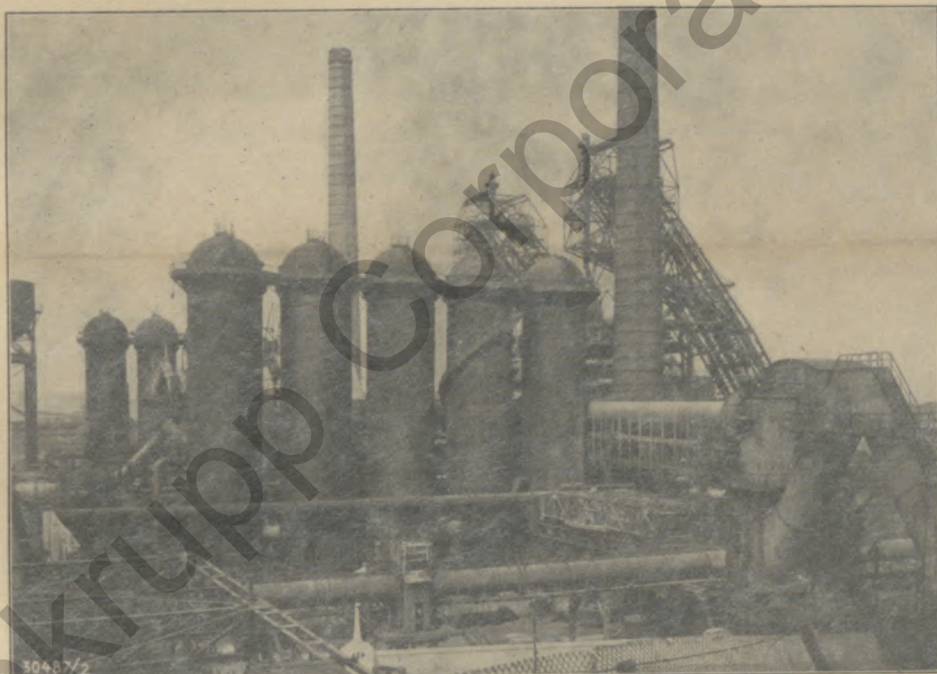
Winderhizer des Hochofens IV
