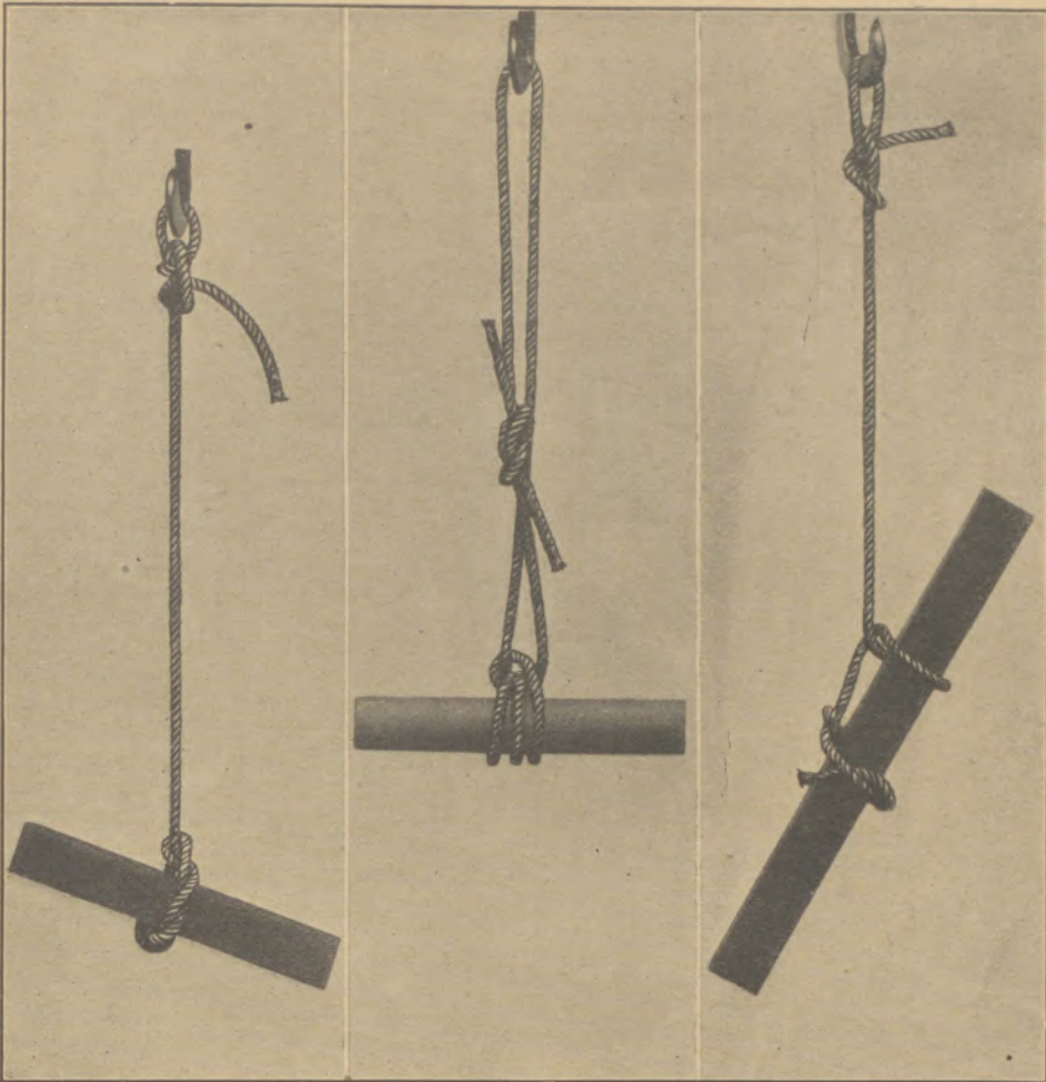
Zimmermannsknoten an der Last, Doppelknoten am Haken für einfaches Seil (z. B. bei Transport un- arbeiteter Hölzer.)
