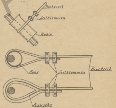
Herstellung von Schlaufen bei Drahtseilen mittels Seilklemmen.
