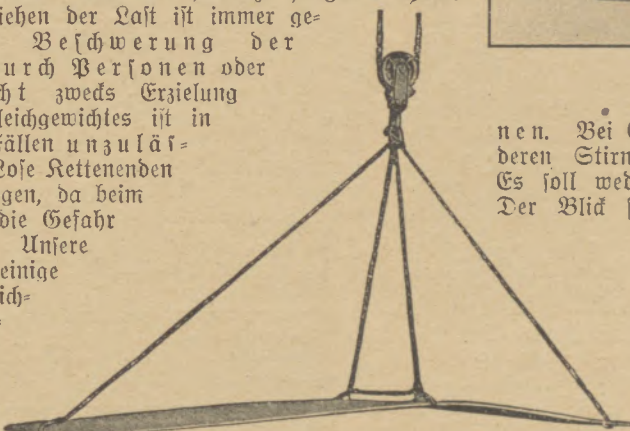
Transport von Platten mittels Anhängen von 4 Ketten.
