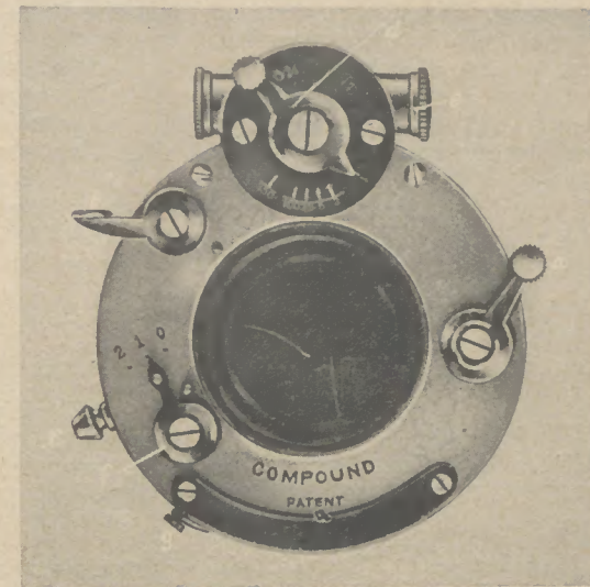
Abb. 5: Compound-Verschluss mit Lufthemmung der Fa. Dedel, München a = Spannhebel, b = Fingerauslöser, c = Nippel für Ballauslösung, d = Einstellzeiger für Belichtungszeit, e = Pumpe für Lufthemmung, f = Einstellzeiger für Zeit und Moment, g = Blendenzeiger
