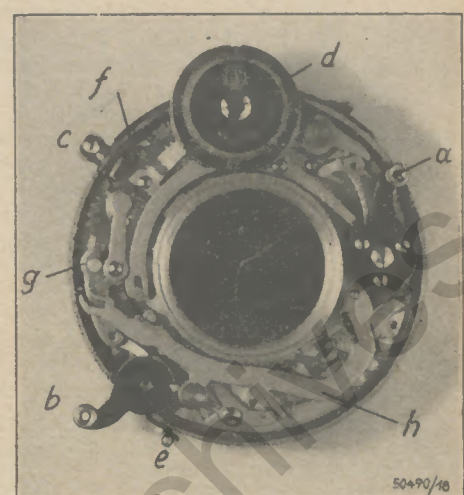
Abb. 6: Compur-Verschluss mit Räderhemmwerk der Fa. F. Dedel, München a = Spannhebel, b = Fingerauslöser, c = Nippel für Drahtauslöser, d = Einstellzeiger, e = Blendenzeiger, f = Räderhemmwerk, g = Hemmwerksanker, h = Schalthebel für Automat- oder Spannverschluss
