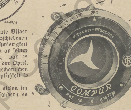
Abb. 7: Compur-Verschluss der Fa. Dedel, München, mit Räderwerks-hemmung und Selbstauslöser a = Spannhebel, b = Fingerauslöser, c = Nippel für Drahtauslöser, d = Stellring für Moment-, Druck- oder Zeitauslösung, e = Blendeneinstellung, f = Knopf für eingebauten Selbstauslöser
