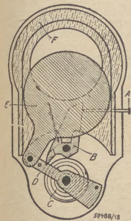
Abb. 2: Zwei-Lamellen-Verschluss von Steinheil in München 1895 D.R.G.M. (konstruiert von Karl Preißner)
