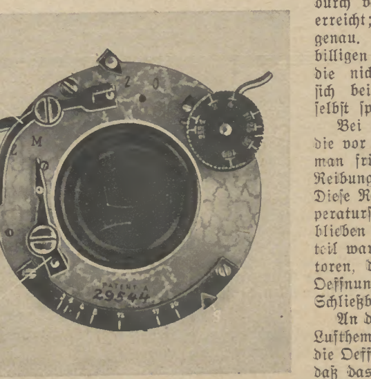
Abb. 4: Verschluss mit Reibungsbremse der Fa. Dedel, München a = Spannhebel, b = Fingerauslöser, c = Auslösepumpe, d = Bremscheibe, e = Zeit- und Momentzeiger, g = Blendenzeiger
