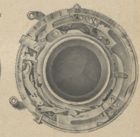
Abb. 8: Compur-Verschluss (wie Abb. 7) mit durchsichtiger Deckplatte
