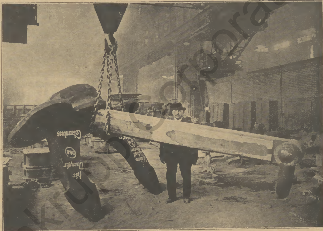
Union-Patentanker von 9750 kg. Gewicht
