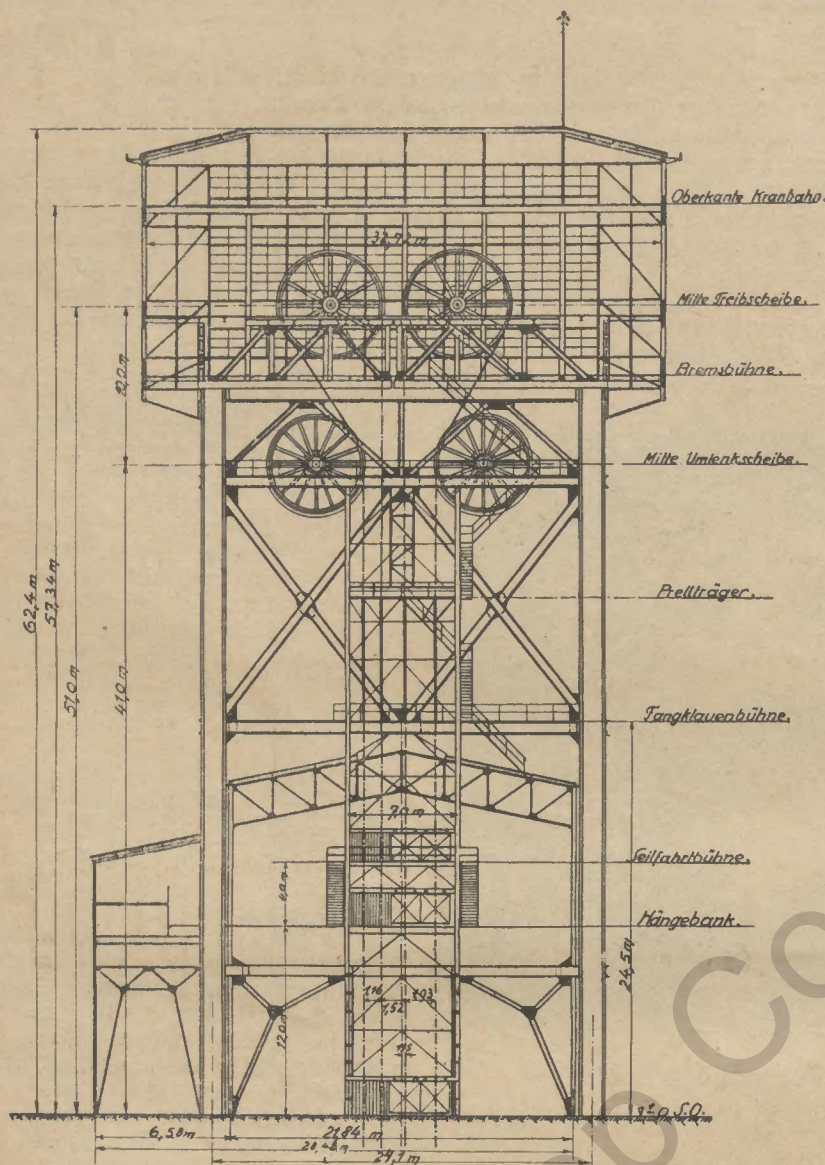
Ansicht des Förderturmes.
