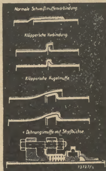
Die gebräuchlichen Schweißverbindungen
