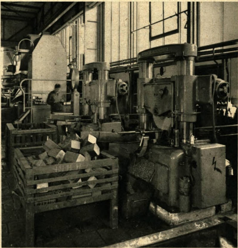
▼ Einen neuen Sägeraum richtete die Schmiedag ein. Im Vordergrund zwei der Öldrucksägen, mit denen man Knüppelmaterial vor der Weiterverarbeitung auf das verlangte Gewicht zurechtsägt
