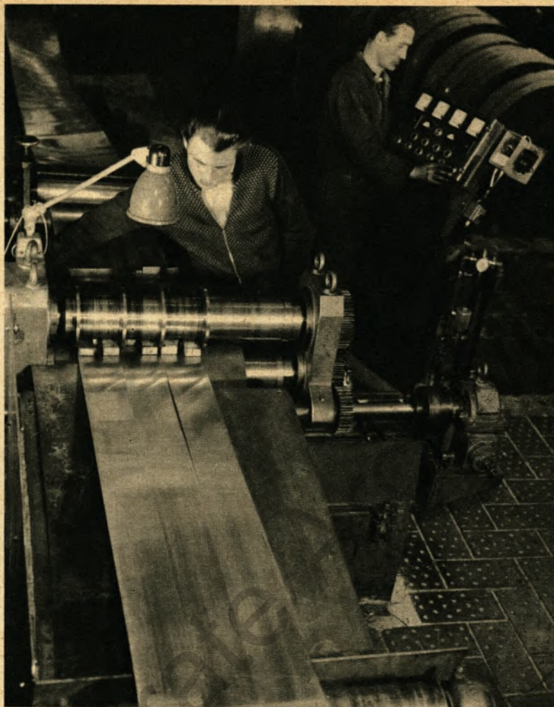
▲ Für die vollkontinuierliche Mittelbandstraße der Hoesch Walzwerke in Hohenlimburg wurde im Berichtsjahr ein zweiter Stoßofen in Betrieb genommen. Diese Mittelbandstraße liefert seit 1955 Qualitätsband, das alle Forderungen nach engsten Toleranzen, sauberster Oberfläche und bester Gefügebildung erfüllt
