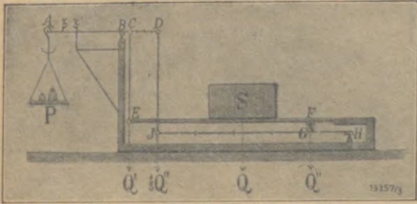
Abb. 5: Brückenwaage
