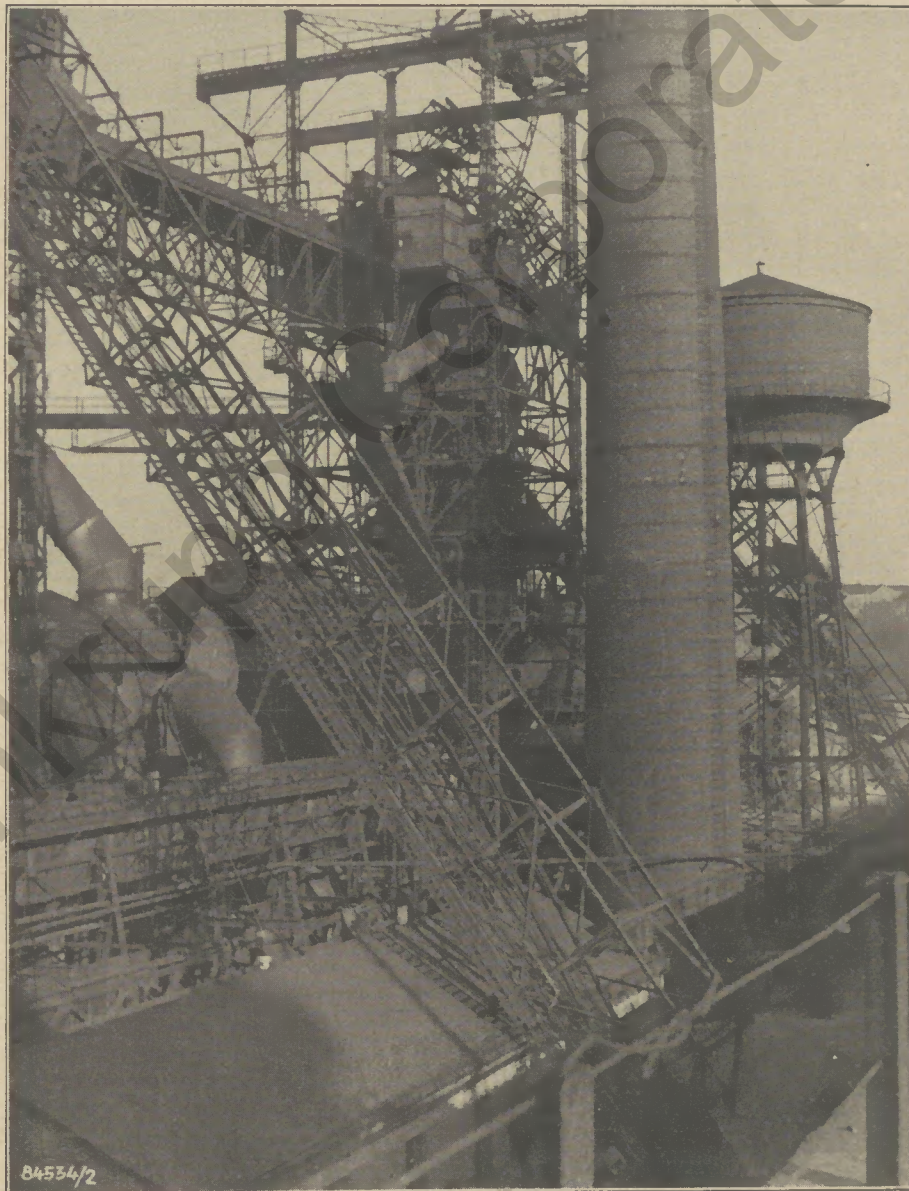
Hochofenanlage mit Schrägaufzügen
