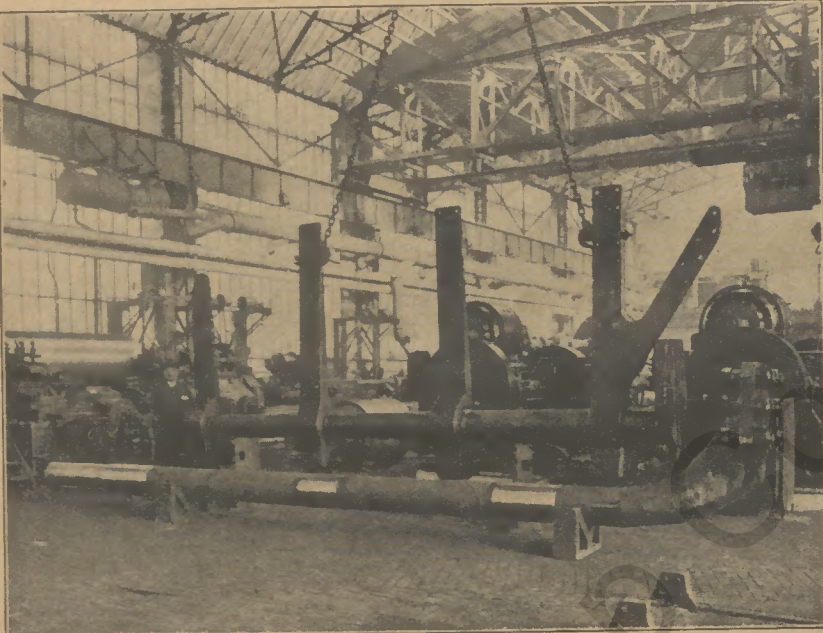
Geschmiedetes Schiffsruder (Ruderschaft und Ruderrahmen) in der Bearbeitungs-werkstatt unseres Hütewerks.
