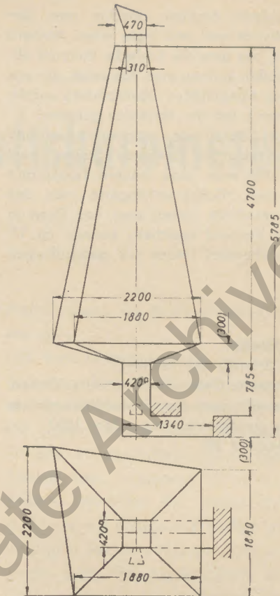
Siegerländer Hochofen mit langem Eck 1607 (6)
