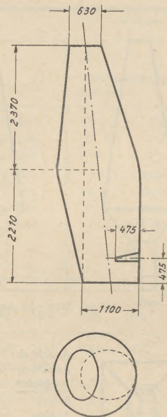
Wendelsteiner Floßofen 1762 (7). Der Gestellquerschnitt ist gegen den Gichtquerschnitt verdreht. Eine Blasform.
