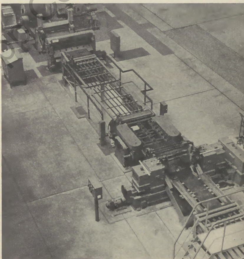
Richtmaschine und Besäumschere in der Linie
