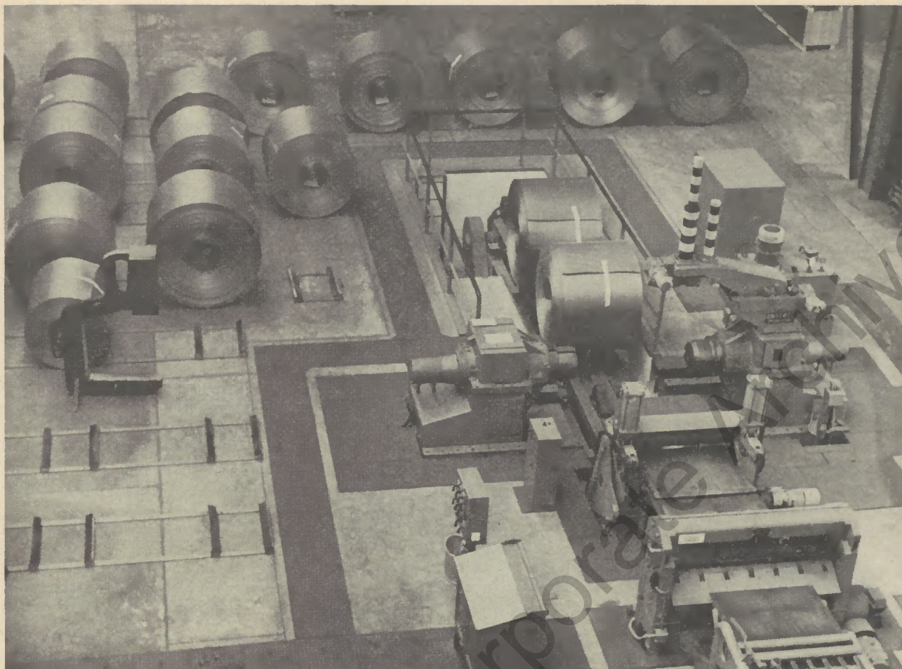
Einlaufteil der Anlage
