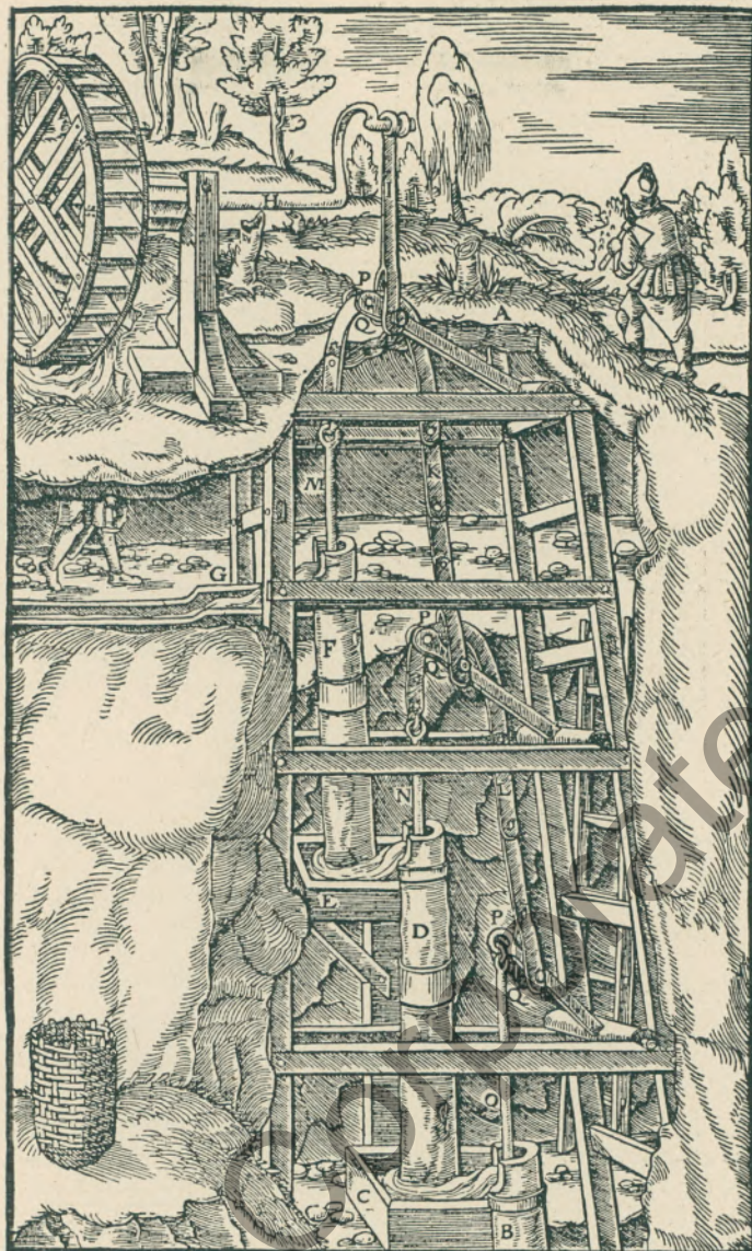
Abb. 7. „Stangenkunst.“ (Aus Agricola, Berg- und Hüttenwesen 1556.)
