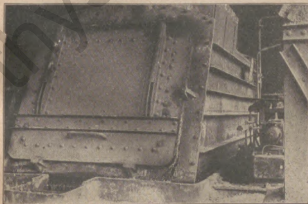
Bild 2: In die Aussparung der Platte wird ein geteerter Asbestzopf eingelegt, der sicher abdichtet und keine Flammenbildung zuläßt
