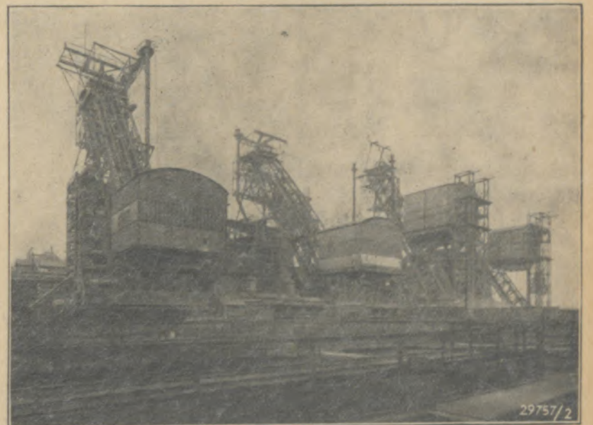
Abb. 7: Gesamtansicht der neuen Hochofenanlage, Ofen 1-4, von der Bunkerseite gesehen
