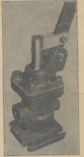
Abb. 7: Sicherung an Hebelsteuerungen
