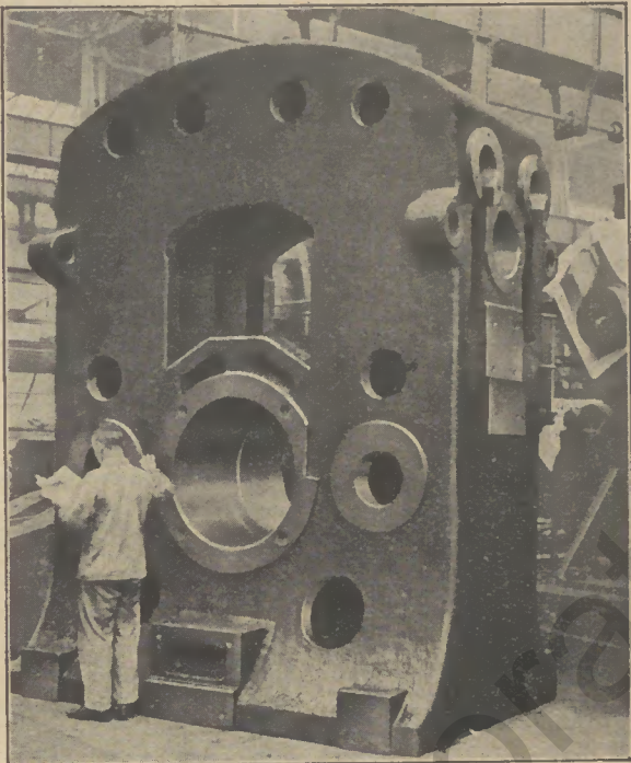
Pressenständer im Gewichte von 44 000 Kg. den wir unter Rom. 749,20 an Maschinenfabrik Meer u. G., München-Glabbach, geliefert haben, hergestellt in unserer Stahlgießerei.
