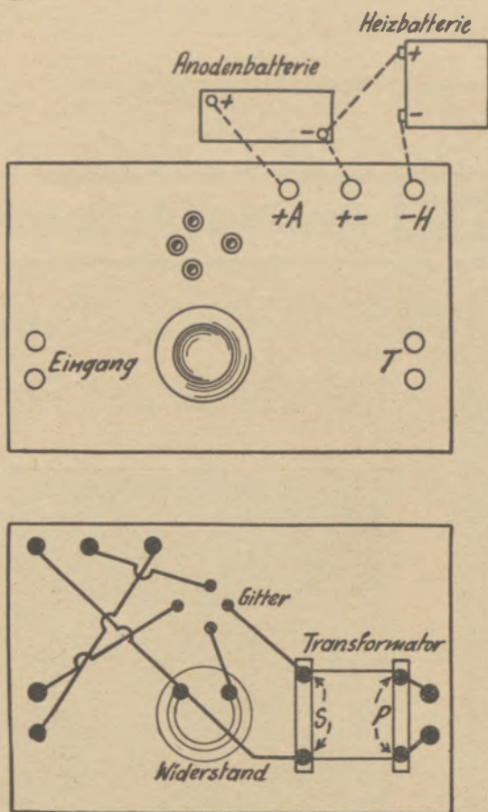
Abb. 2: Bauzeichnung des Verstärkers.
