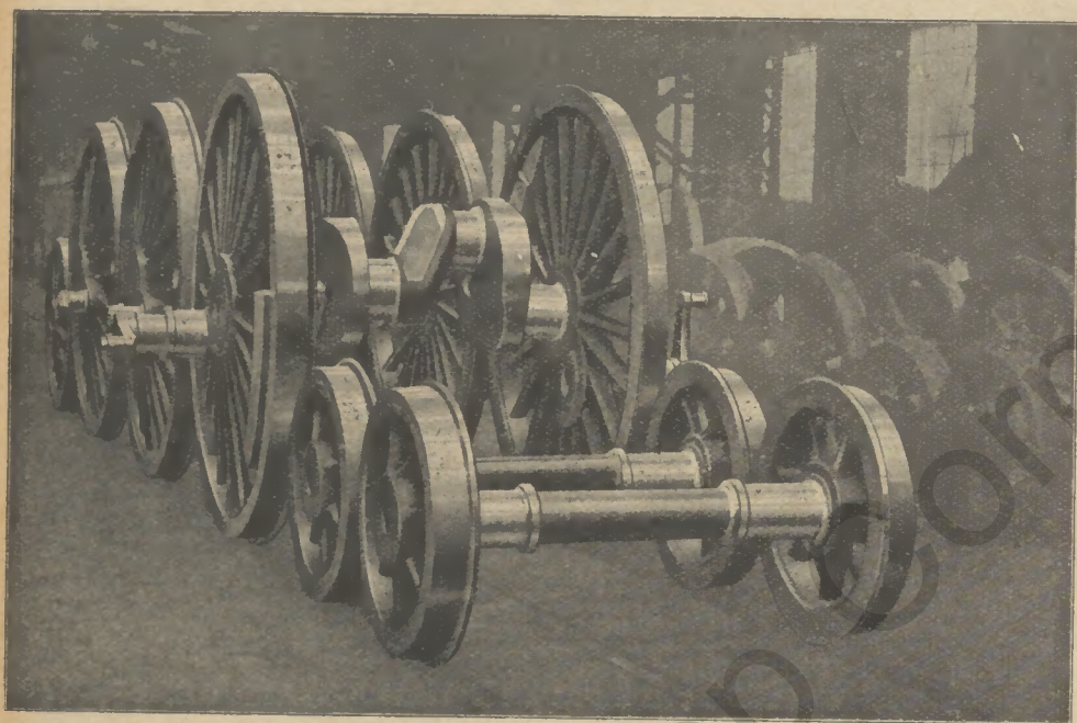
Unten: Aus unseren Radsatzwerkstätten: Radsätze mit Zahnrädern
