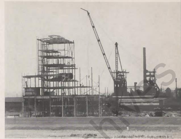
Das Stahlskelett der Sinteranlage: Gegenwärtig entsteht auf dem durch die Ruhrverlegung gewonnenen Hüttengelände der Stahlbau der Sinteranlage, die voraussichtlich Mitte 1961 fertiggestellt sein wird. Sie soll in der Lage sein, monatlich 40 000 t Sinter für unsere Hochöfen zu erzeugen. Im Verlauf des Sinterprozesses werden Feinerze (Korngröße unter 1 mm), die normalerweise schlecht verhüttbar sind, in stückige Form umgewandelt, und dadurch eine wirtschaftliche Verhüttung ermöglicht (vergl. WZ 12/59).
