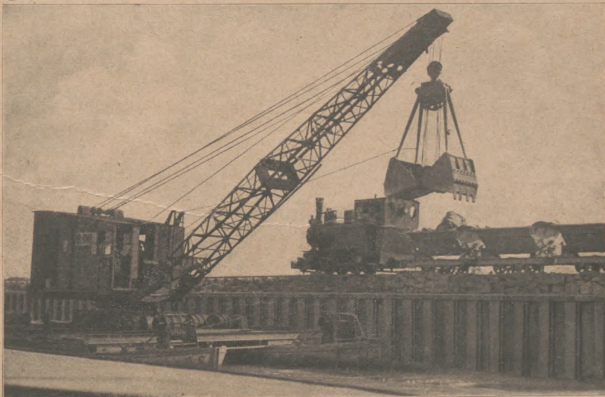
Auf viele Kilometer Länge wurden Larssenbohlen gerammt. Das Bild zeigt den Aushub der alten Kanalböschung vor der Wand. Der Boden wird zur Hinterfüllung der Spundwand teilweise wieder verwendet
