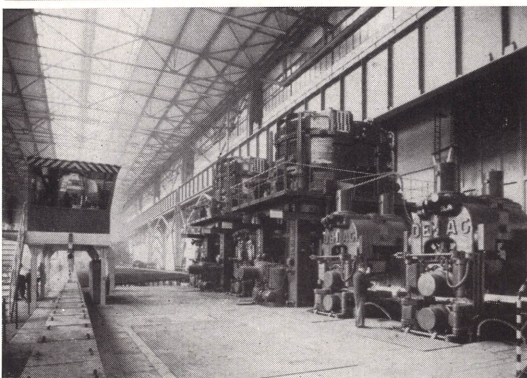
Halbzeugstraße
