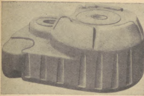
Bild 4 Kern aus kalthärtendem Kunstharz
