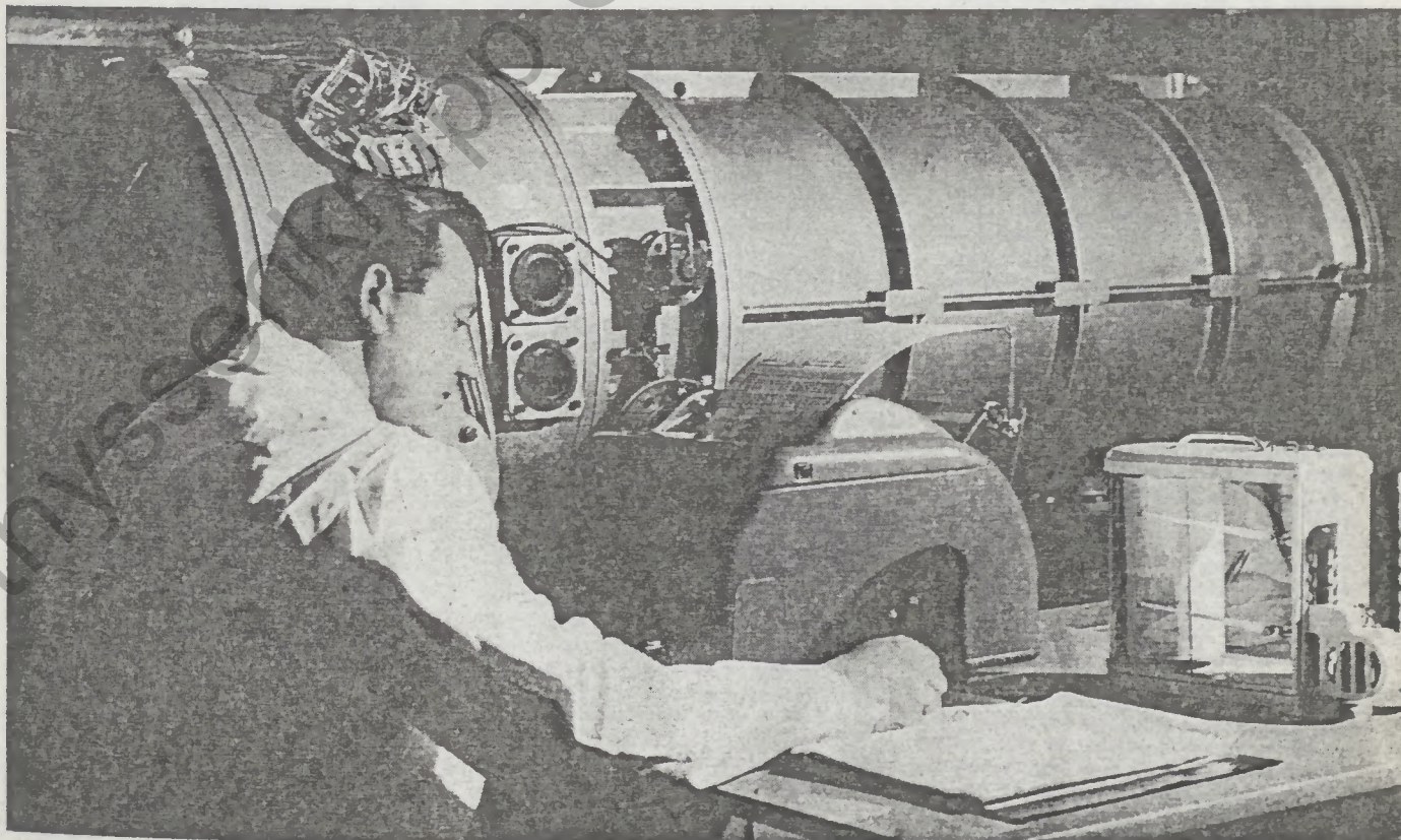
Ankunft der Resultate in der Fernschreib-Ausgabemaschine. Im Hintergrund der Vakuum-Kessel des Spektrometers
