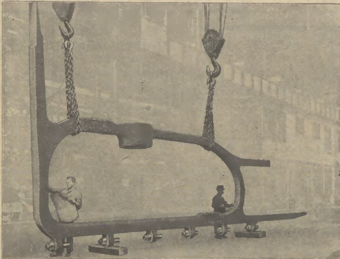
Fertigbearbeiteter Schiffshintersteben im Gewicht von ca. 21 500 kg
