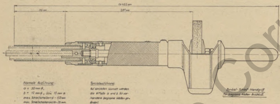
Bild 1. Dynbalhandgriff mit federnder Lagerung.
