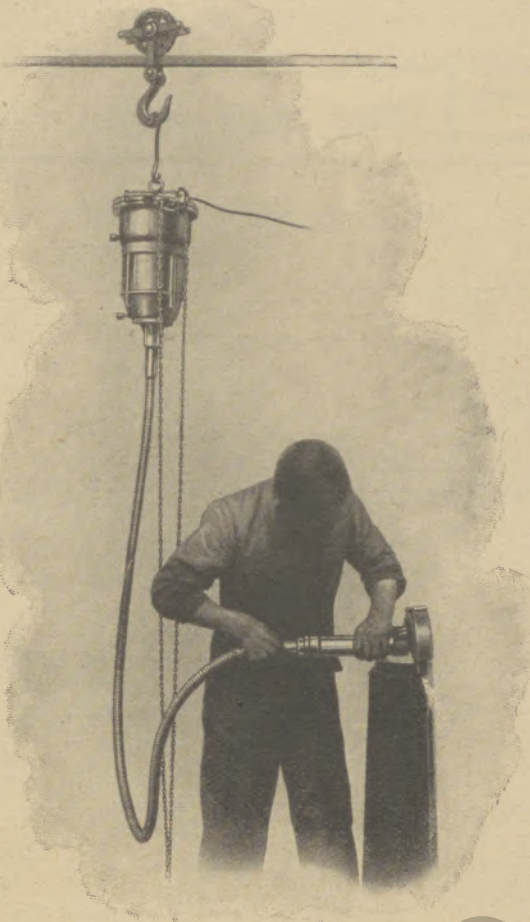
Bild 3. Hängende Dynbal-Schleifmaschine.
