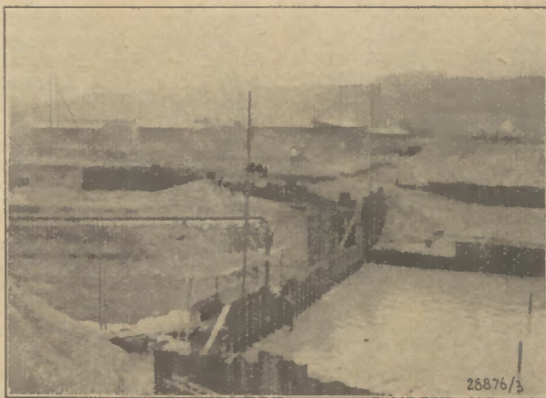
Vertwendung von Larsseneisen der Dortmunder Union bei Wasserbauten an der Iller im Allgäu (Aufnahme von Hans Baer, Dortm. Union, C 21)
