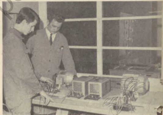
Bild 2: Der Motorenstand kann durch Steckverbindungen mit anderen Prüf- und Meßeinrichtungen verbunden werden und hilft schaltungstechnische Zusammenhänge richtig zu verstehen.
