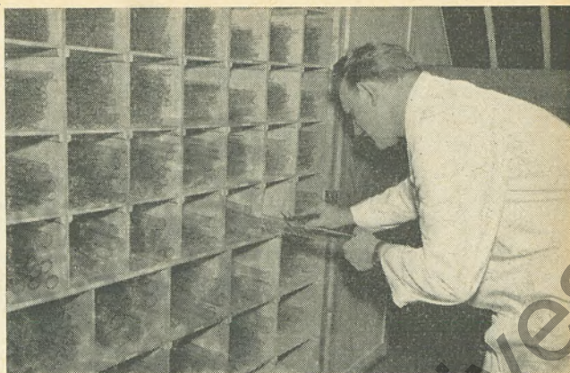
Alle hier im Röhrenregal vereinigten Röhre sind 1,50 Meter lang
