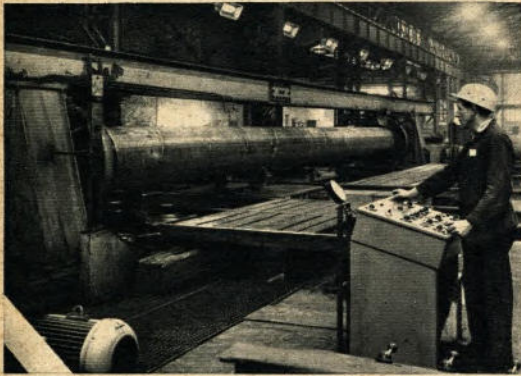
▲ Jedes Rohr wird durch hohen Wasserdruck auf Dichte und Festigkeit geprüft, Horst Krüger am Steuerpult
