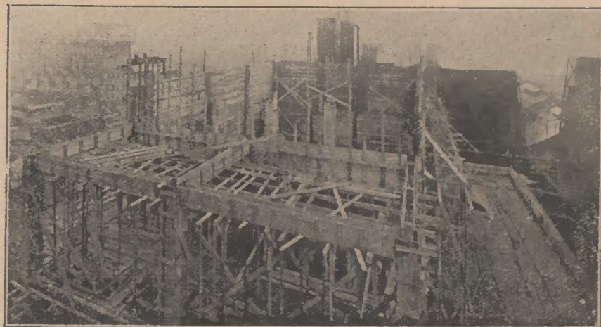
Arbeiten am Koksstapelbunker 1. Dezember 1926. Von Koks-enturm III aus gesehen.
