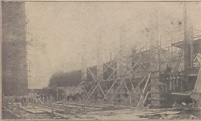
Betonierung der Vorkläranlage. Mit der Aufstellung der Säulenschalung für den Löschurm wird begonnen.
