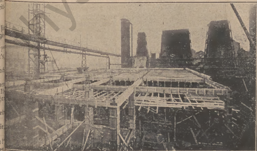
Arbeiten am Koksstapelbunker im November 1926.
