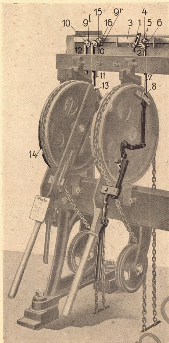
Abb. 13 Wirkung der Handfalle am Stellhebel
