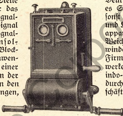
Abb. 8 Blockapparat mit Konsolwinde
