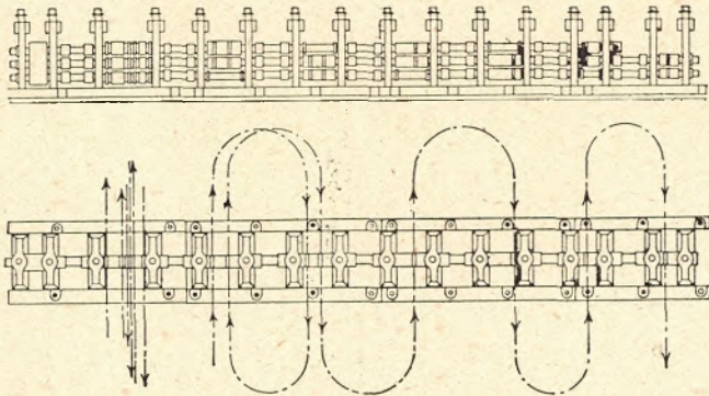
Abb. 1 Belgische Drahtstraße
