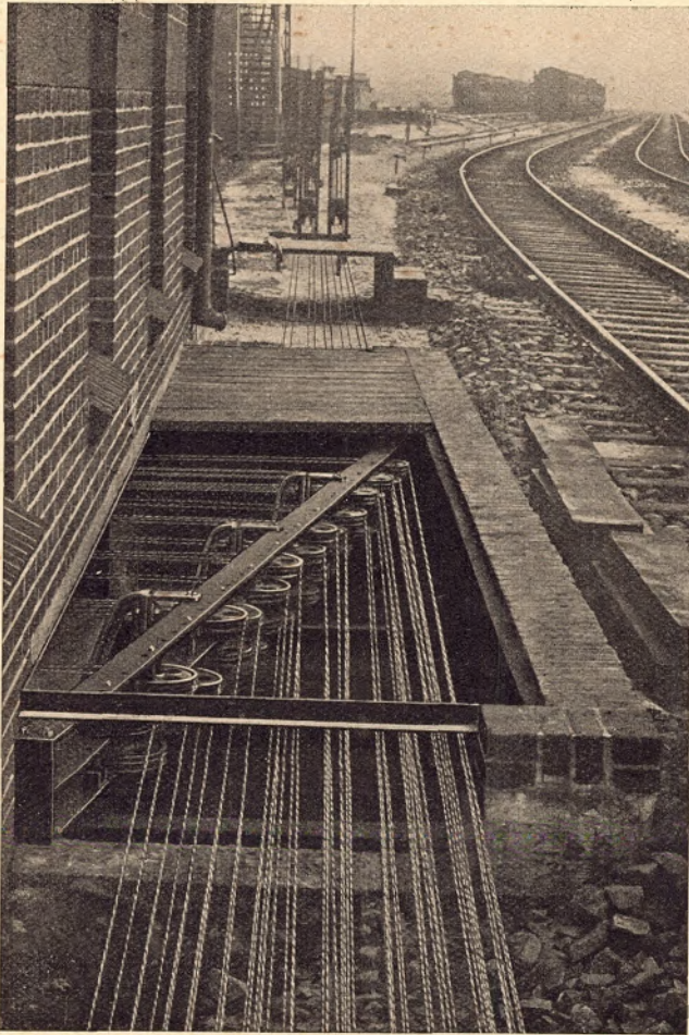
Abb. 10 Drahtumlenkungen in einem neueren mechanischen Stellwerk
