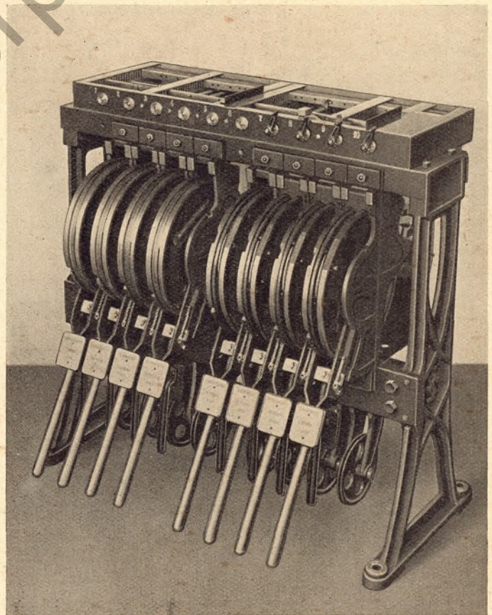
Abb. 12 Schieberkasten über dem Hebelwerk eines Siemensschen mechanischen Stellwerkes (Blockkasten abgenommen)
