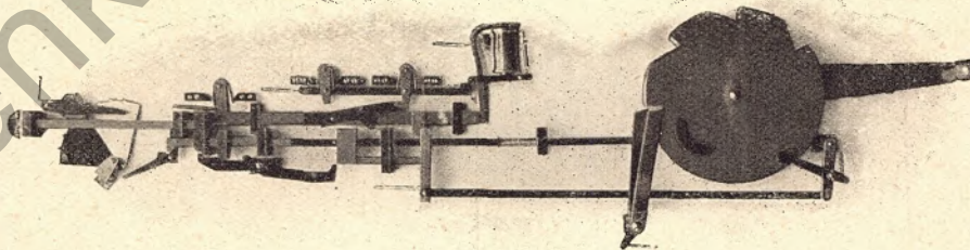
Abb. 9 Blockverschuß eines Signalhebels durch ein Blockfeld
