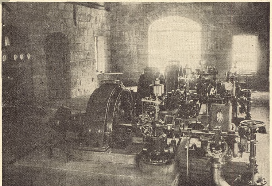
Abb. 3. Wasserkraftanlage Incachaca (Bolivien), 2300 Meter über Meereshöhe. Maschinenhaus
