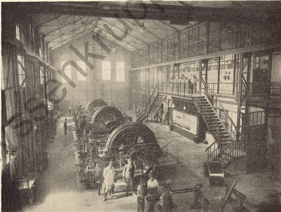
Abb. 1. Siemens-Zentrale mit Dieselmotoren des Salpeterwerks „Chile“, Deutsche Salpeterwerke Taltal
